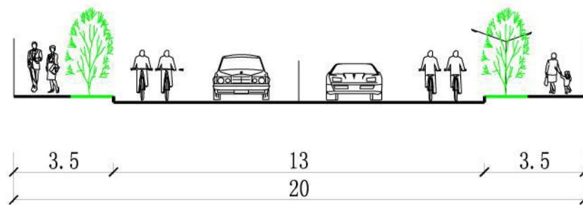
图 1 赣江路道路横断面图
