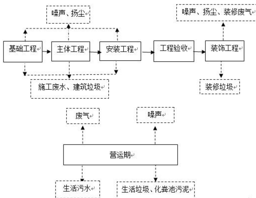
图 3 工艺流程及产污环节示意图
