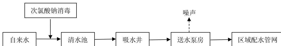
图 1 工程工艺流程及产污环节图
