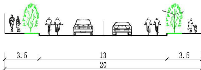
图 1 沅江路道路横断面图
