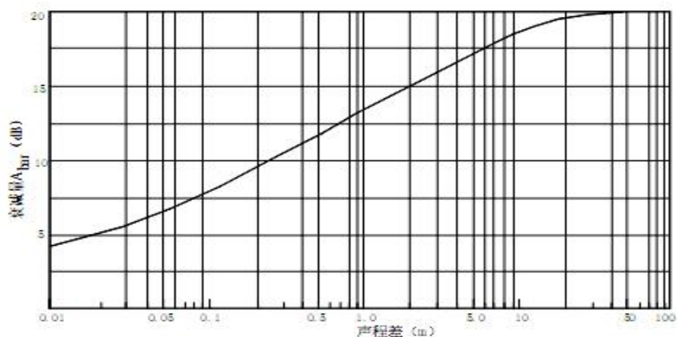
图 7 噪声衰减量 A_{bar} 与声程差 \delta 关系曲线
