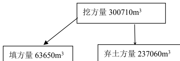
图 3 项目土方平衡图
