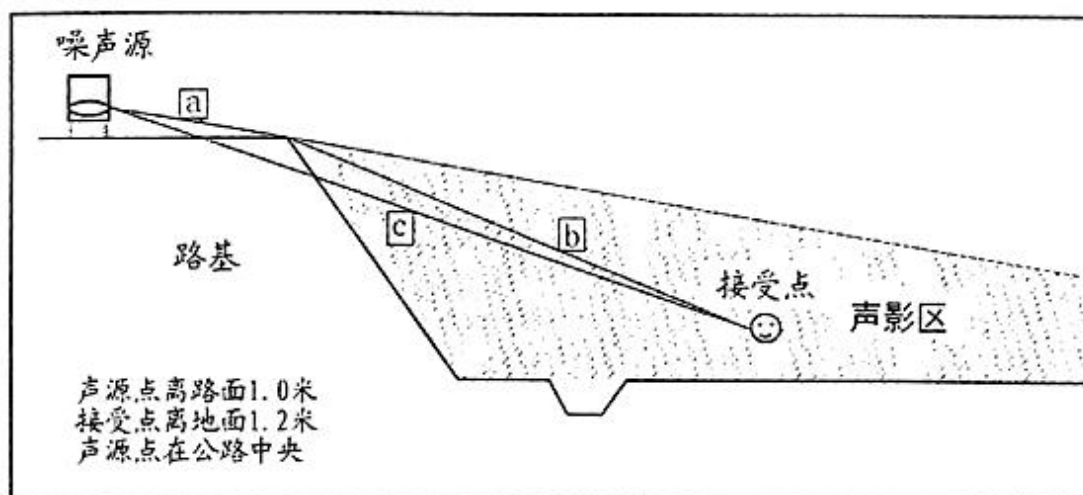
图 6 声程差 \delta 计算示意图
