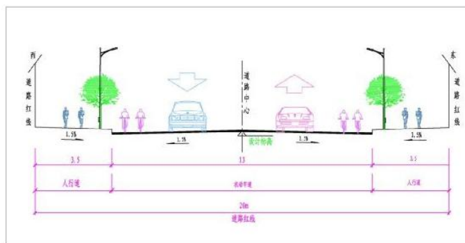
图 1 项目横断面设计图
