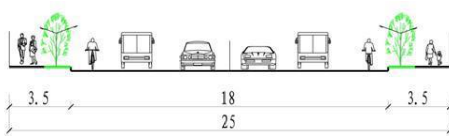
图 1 项目横断面设计图
