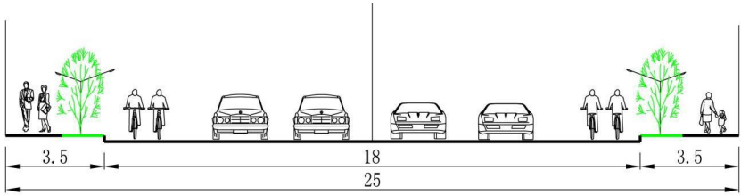
图 1 项目横断面设计图
