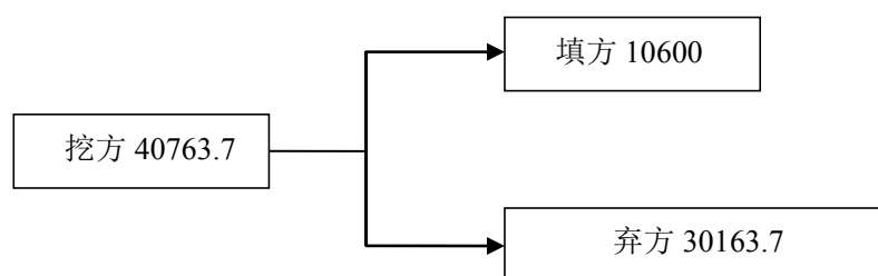
图 2 土石方流向图单位： \text{m}^3
