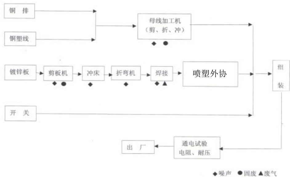
图 2 项目工艺流程及产污环节图
