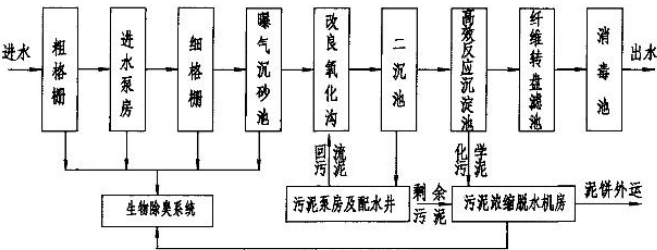
图1 马寨污水处理厂处理工艺
