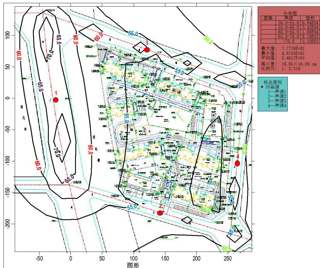
图 5 交通噪声影响分析图
