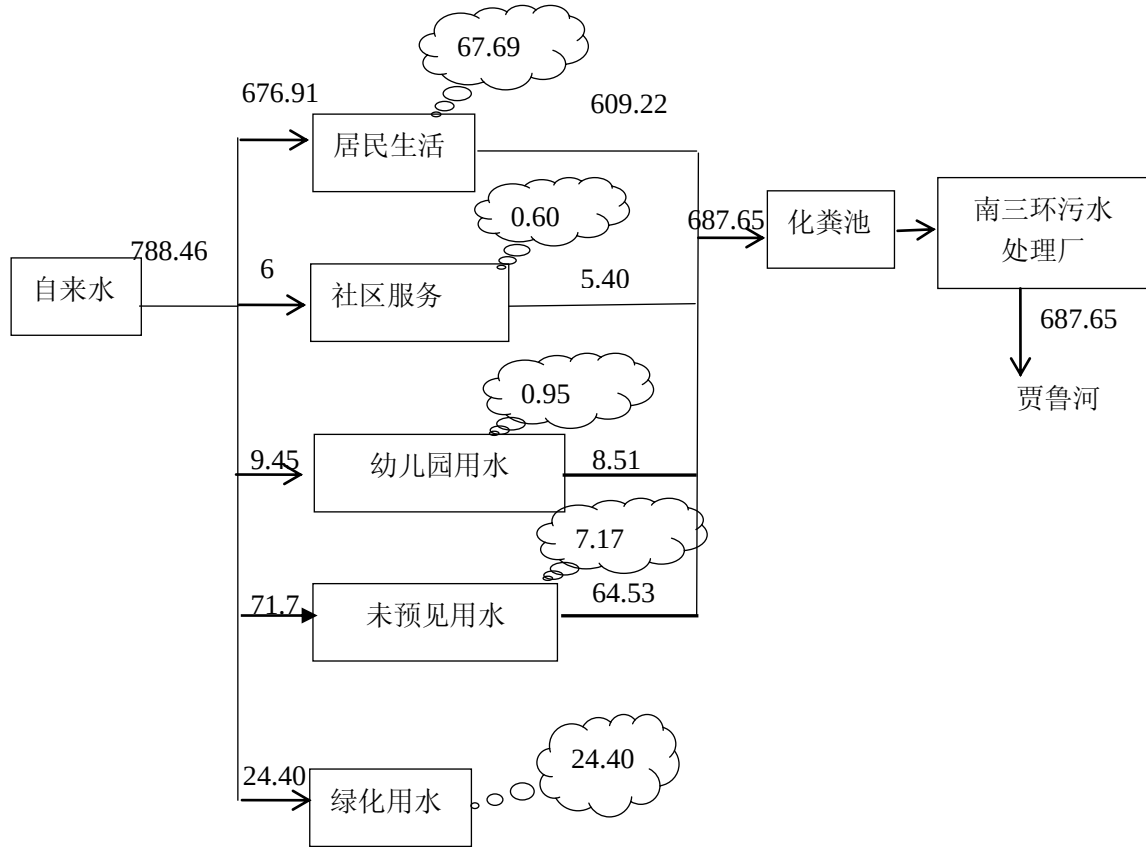
图 4 本项目水平衡图（单位：m 3 /d）
