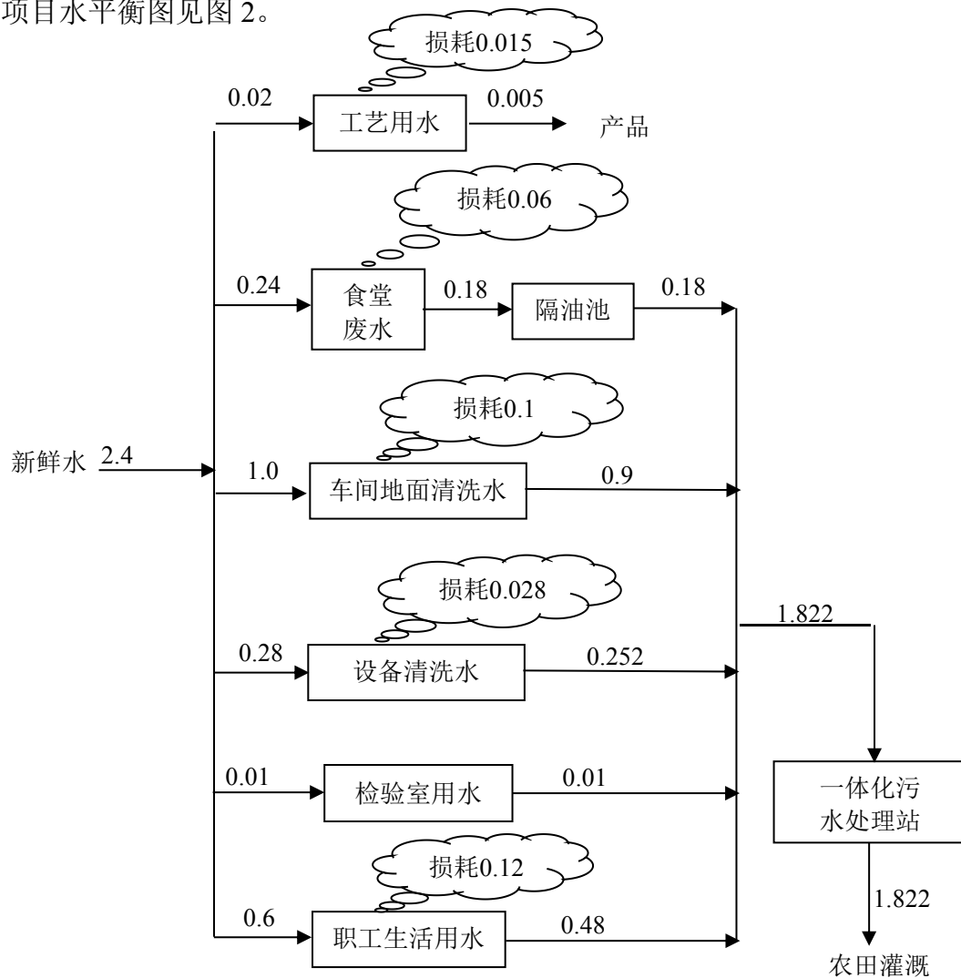
图 2 项目水量平衡图 单位: \text{m}^3/\text{d}
