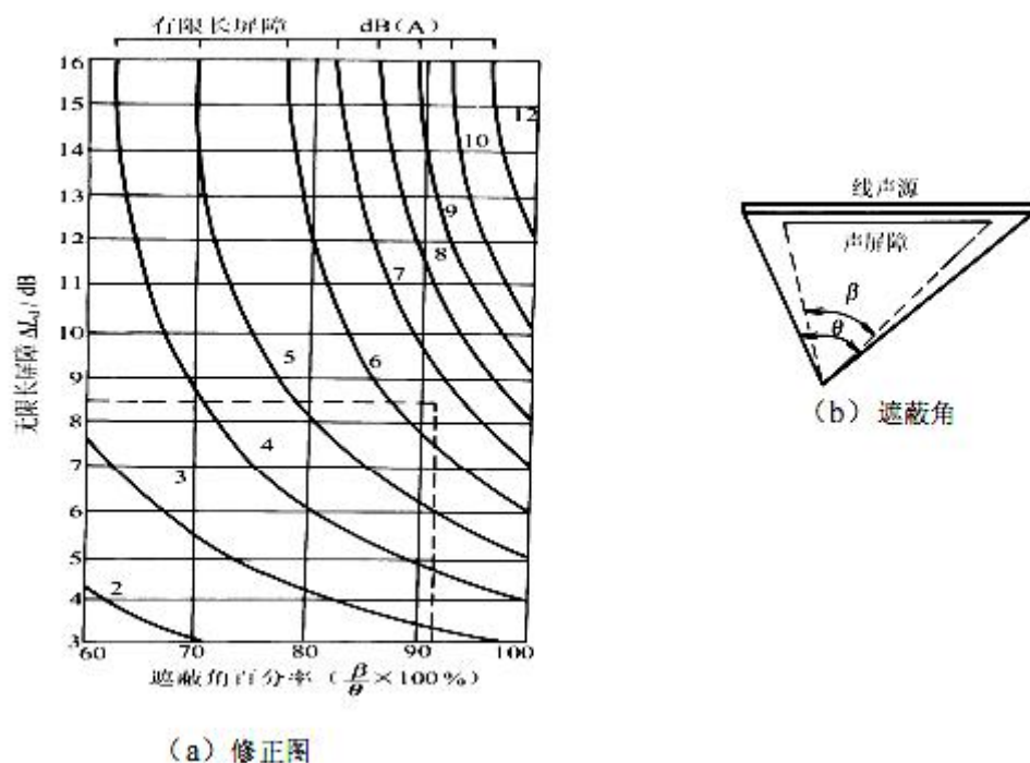
图 5 有效长度的声屏障及线声源的修正图
