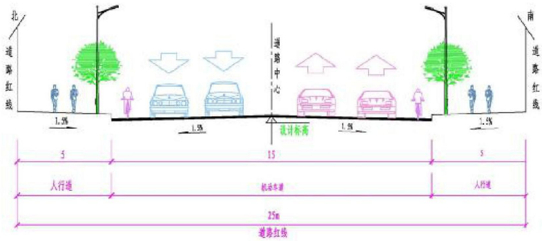
图 1 项目横断面设计图
